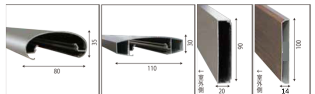
楕円手摺 平手摺 アルミ色 木目色
