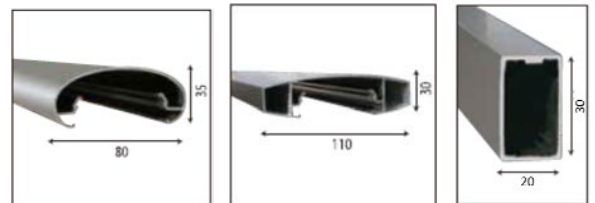
楕円手摺 平手摺
